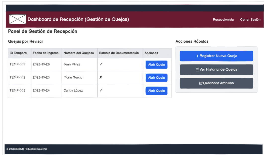
Figura 21: MA-04: Panel de gestión de recepción (Dashboard).
